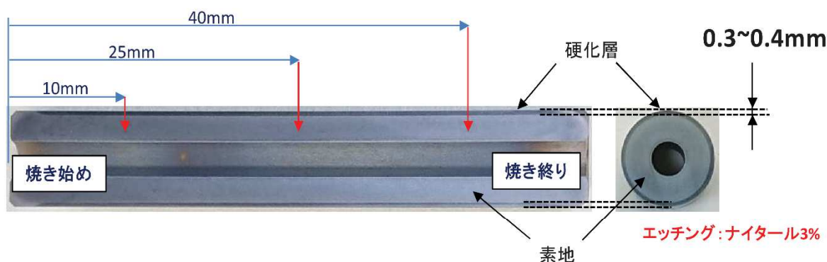
Fig.3 試験材料を縦割りした断面と硬さ測定位置
